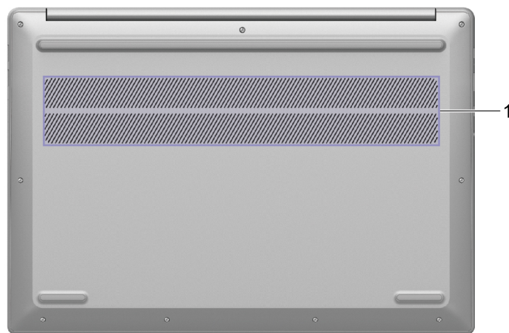
Abbildung 7. Ansicht von unten für 16-Zoll-Modelle (IdeaPad Slim 5 16AHP9, IdeaPad Slim 5 16IMH9 und IdeaPad Slim 5 16IRU9)
