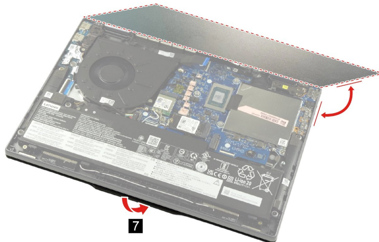
Figure 30. Remove the display module
