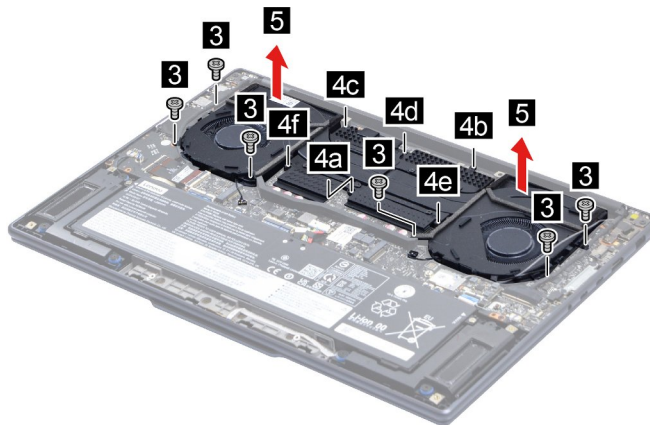
Figure 18. Remove the thermal module
